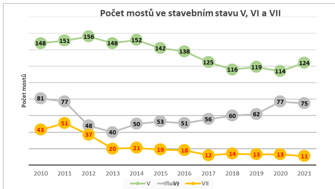
Graf: Počty mostů ve stavebních stavech V, VI a VII
